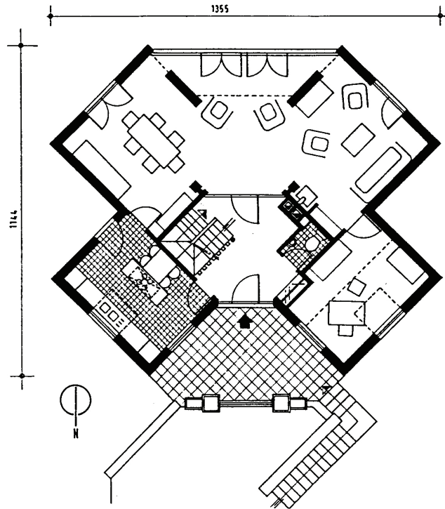
PLAN REZ-DE-CHAUSSEE GELIJKVLOERS
