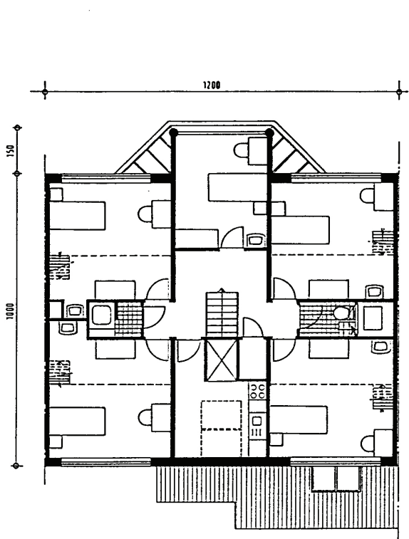
PLAN 1 er ETAGE 1 ste VERDIEPING
